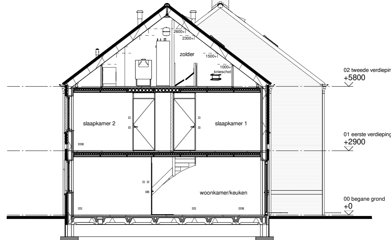
Doorsnede B
