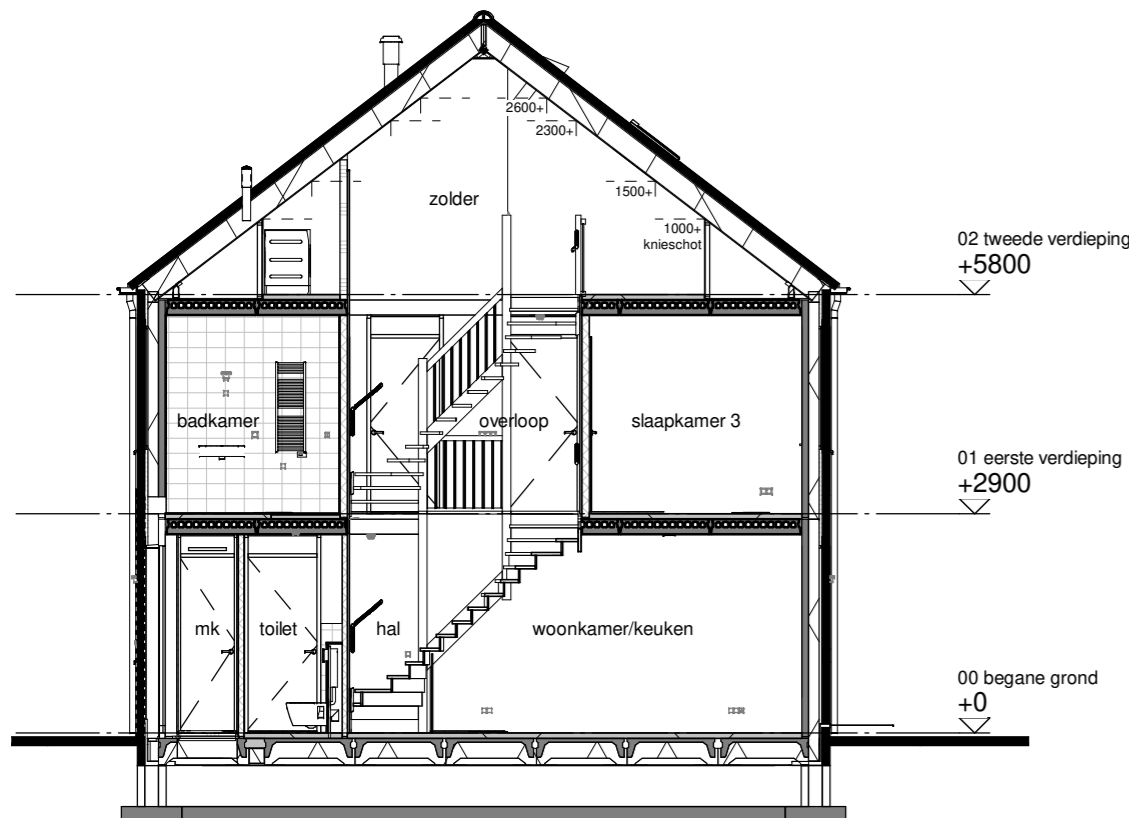
Doorsnede A
