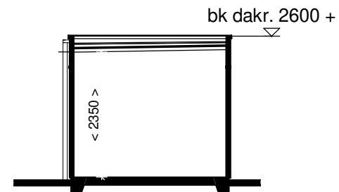
Doorsnede A.
