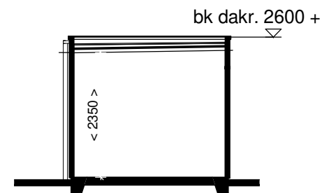
Doorsnede A
