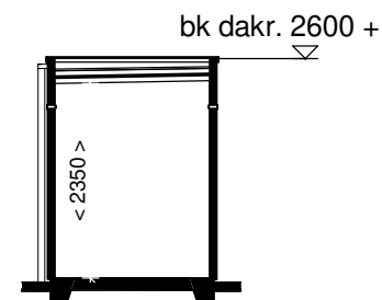
Doorsnede A
