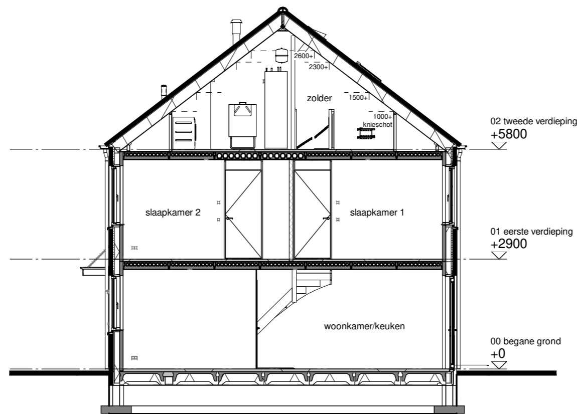
Doorsnede B
