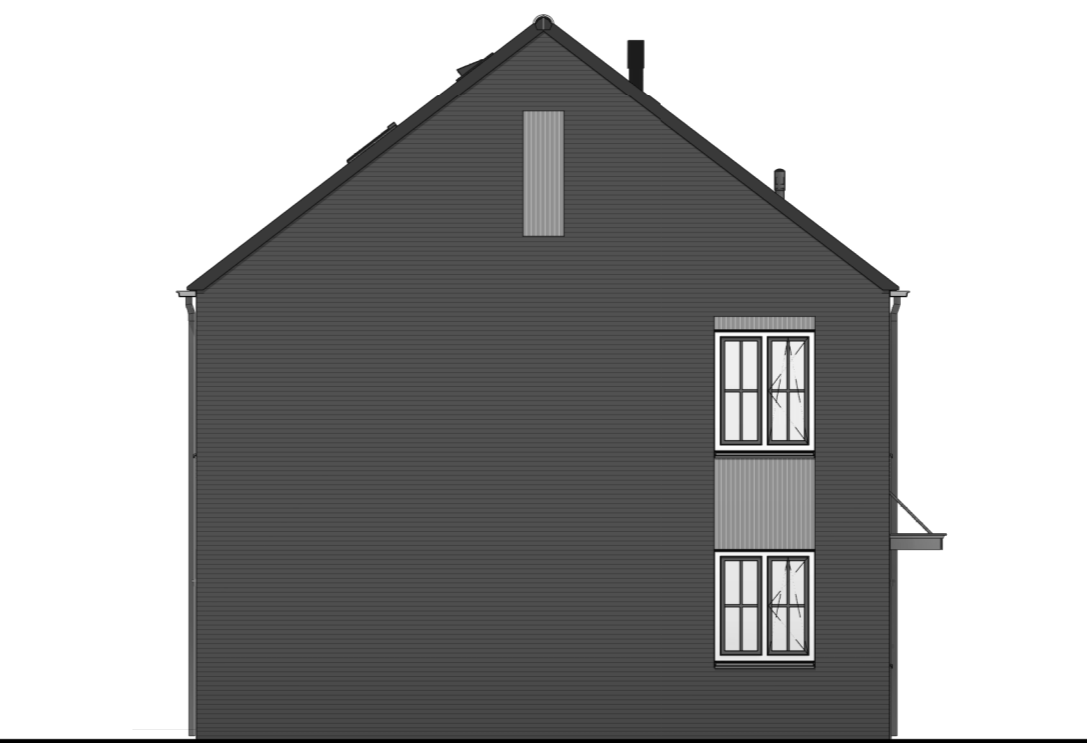
Linker zijgevel
