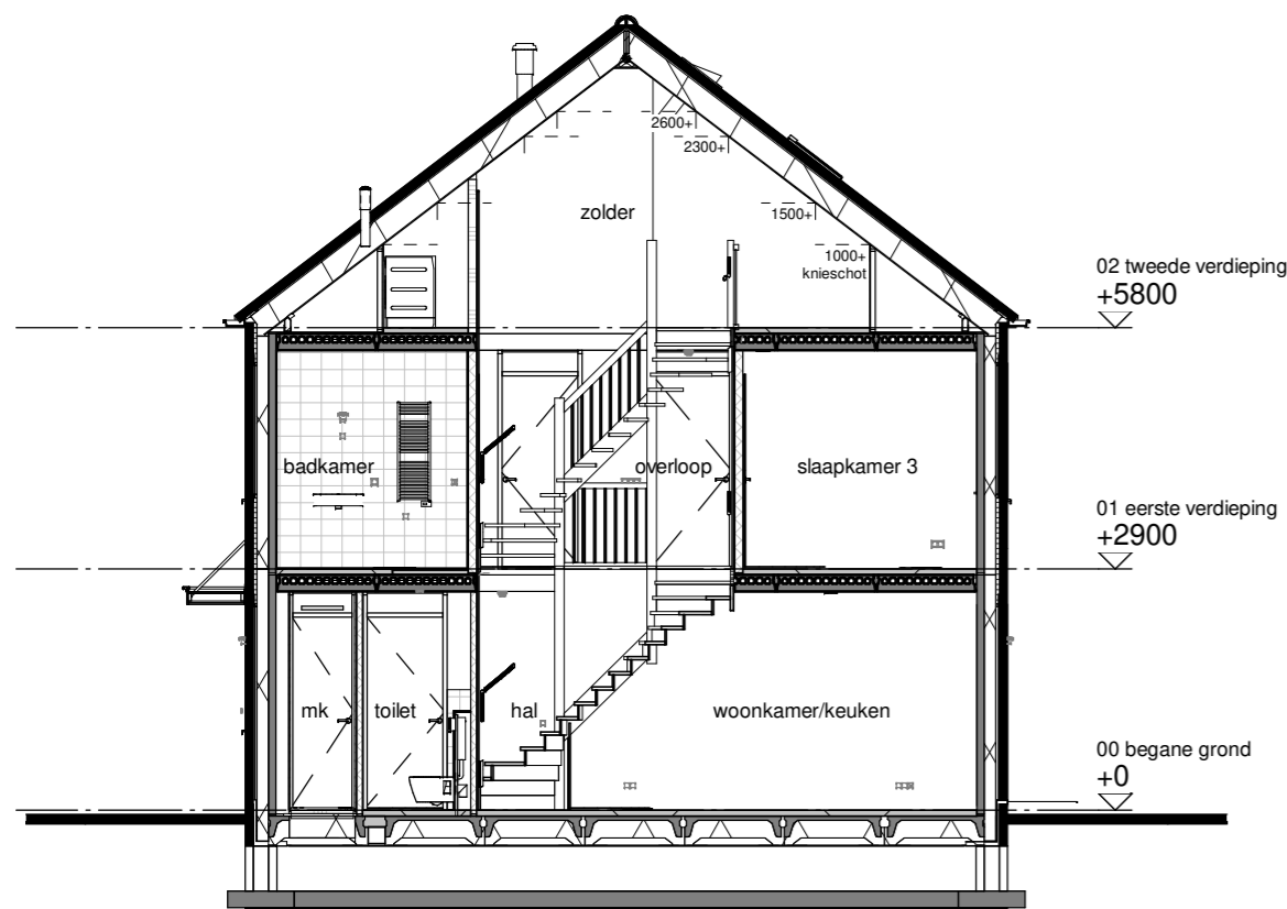
Doorsnede A
