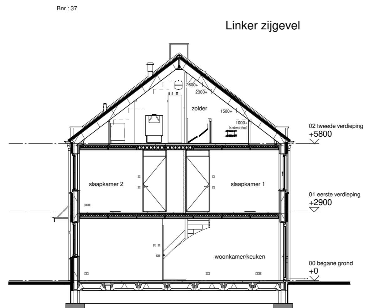
Doorsnede B
