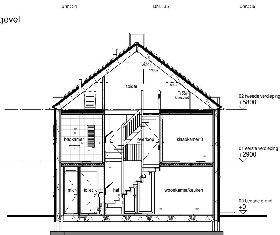
Doorsnede A
